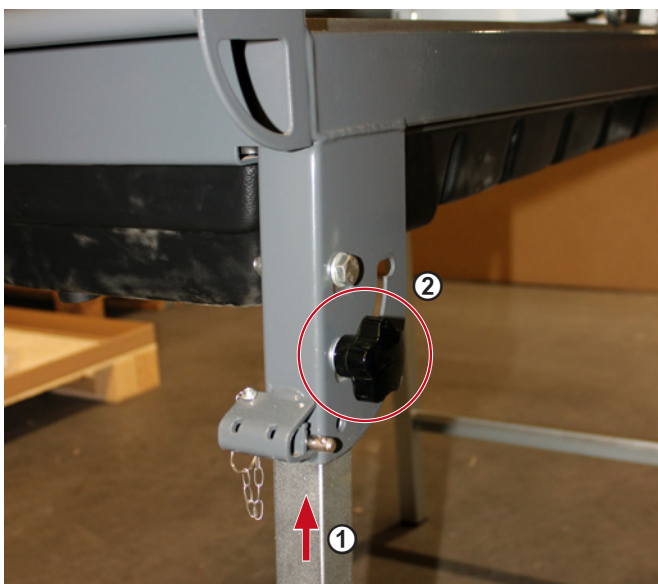
Standfüße hinten einrasten, Kreuzgriffschrauben festziehen Bild 4.9
