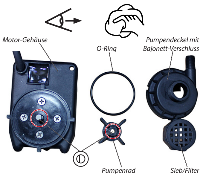
Wasserpumpe demontiert
