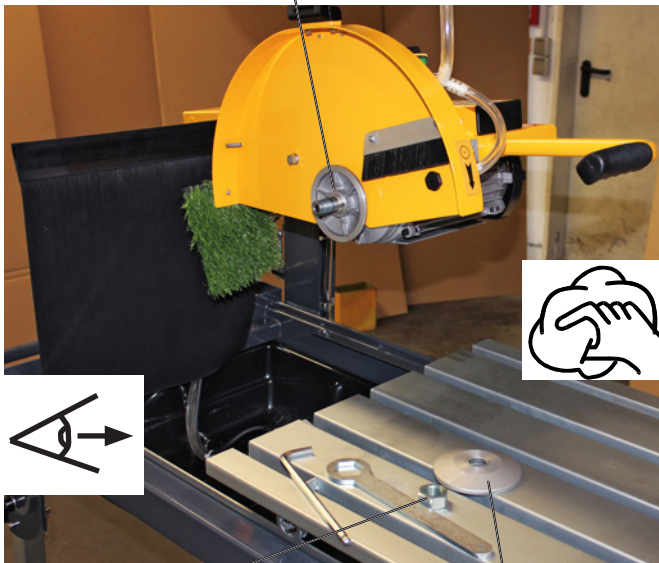
Schneidwellen-Mutter und Druckflansch demontieren Bild 4.19
