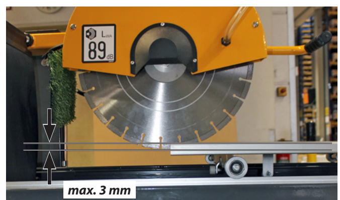
Pendelschneidarm (Trennscheibe) auf die maximale Schnitttiefe eingestellt Bild 4.24
