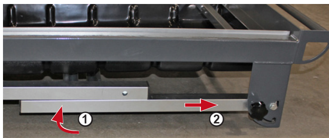
Standfuß austrasten
