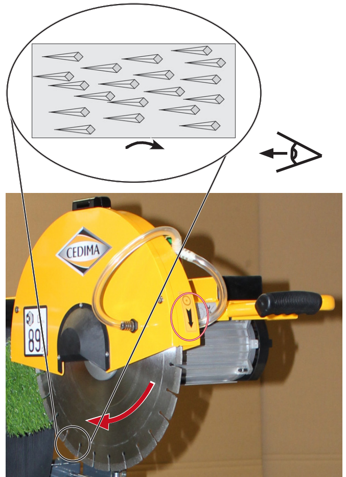
Diamant-Trennscheibe mit der Schneidrichtung der Diamant-Segmente entsprechend der Drehrichtung der Schneidwelle montieren Bild 4.21
