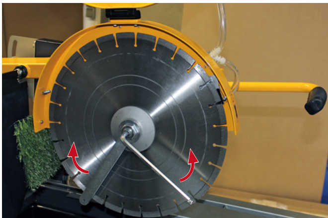
Diamant-Trennscheibe auf die Schneidwelle setzen, Druckflansch mit der Schneidwellen-Mutter an die Diamant-Trennscheibe spannen Bild 4.20
