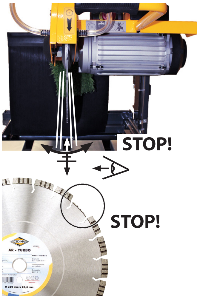
Defekte, flatternde, unrund laufende Diamant-Trennscheibe mit fehlenden Segmenten wechseln
