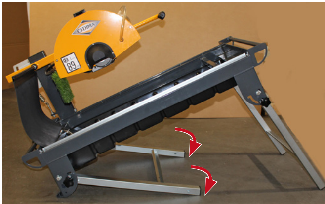
Zweites Standfuß-Paar austrasten und abschwenken Bild 4.8
